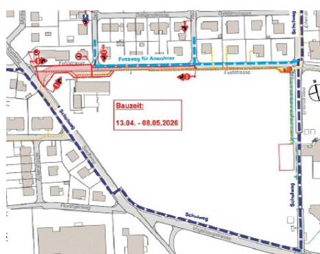
Etappe 2: Leitungen Nelkenstrasse – Rosenstrasse, Parallel Bohrarbeiten am Stadtweg
