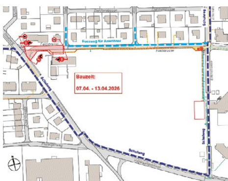
Etappe 1: Leitungen Stadtweg – Nelkenstrasse
